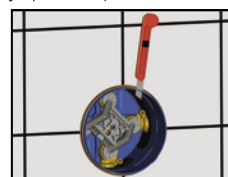
Обрежьте выступающую часть по круговой насечке, отключите воду и демонтируйте устройство промыва.
