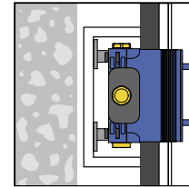
Установка перед стеной на раме
