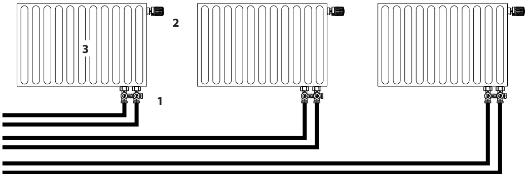
лучевая (двухтрубная) система (байпас закрыт)
